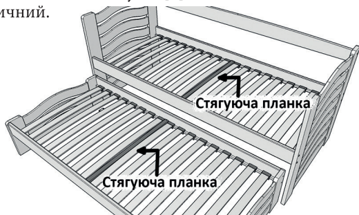
4. Монтаж ламелей
